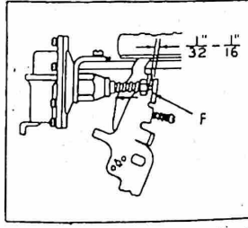
DASHPOT ADJ. Fig.7
