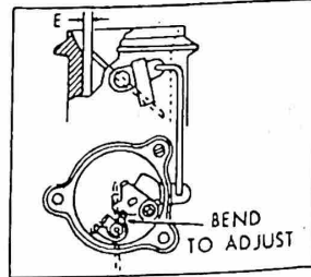
UNLOADER ADJ. Fig.6
