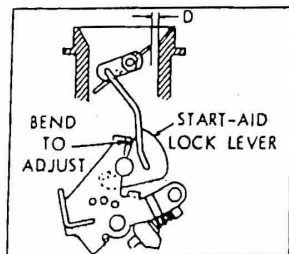
UNLOADER ADJ. Fig.5
